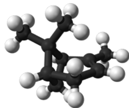
Abb.: Zirben-Geruch Strukturformel C 10 H 16
