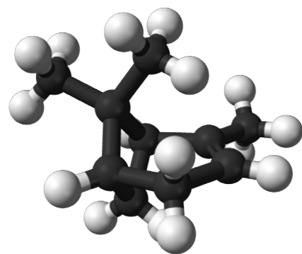
Abb.: Zirben-Geruch Strukturformel C 10 H 16
